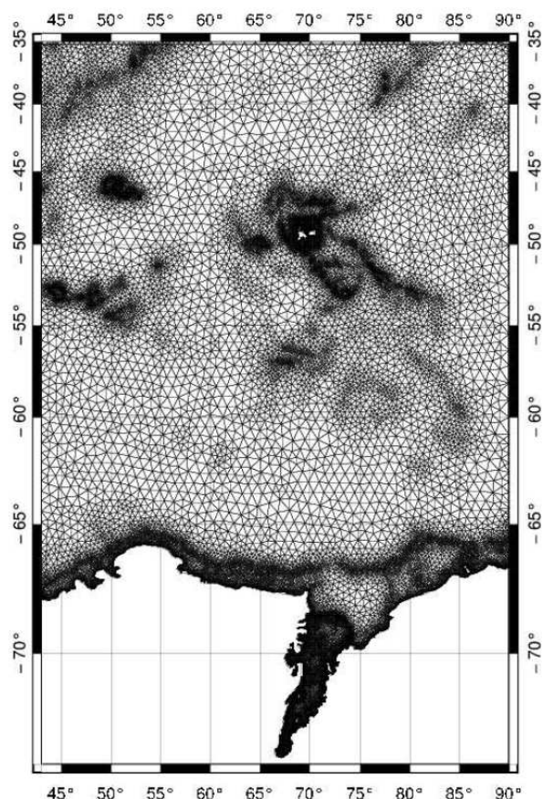
Figure 1. Maillage éléments finis utilisé pour la simulation de la marée
